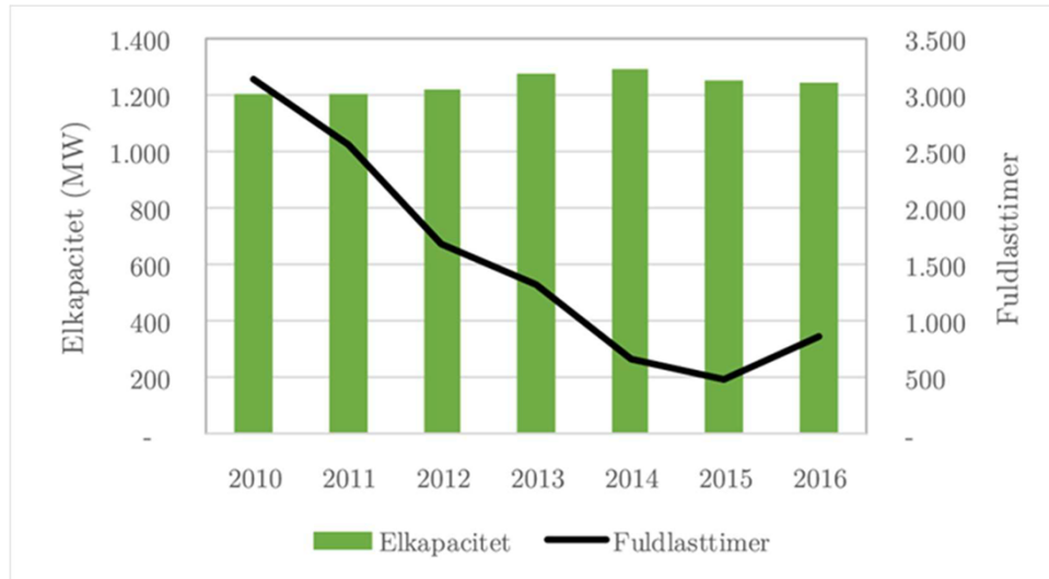
Figur 1 – oversigt over udvikling i driftstimer for gas-generatorer fra ForskEL-rapporten.
