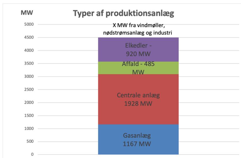
Figur 8 - Reservekraftkapacitet i DK1.
