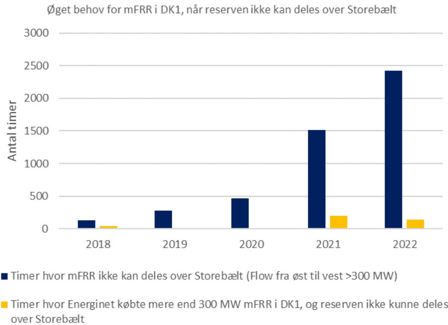
Figur 4: Energinets opkøb af mFRR i timer, hvor 300 MW reserve ikke kan deles fra DK2 til DK1. Kilde: Energinet.
