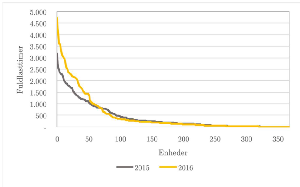
Figur 2 – årligt antal driftstimer fordelt på 350 kraftvarmeværker- oversigt fra ForskEL-rapporten.
