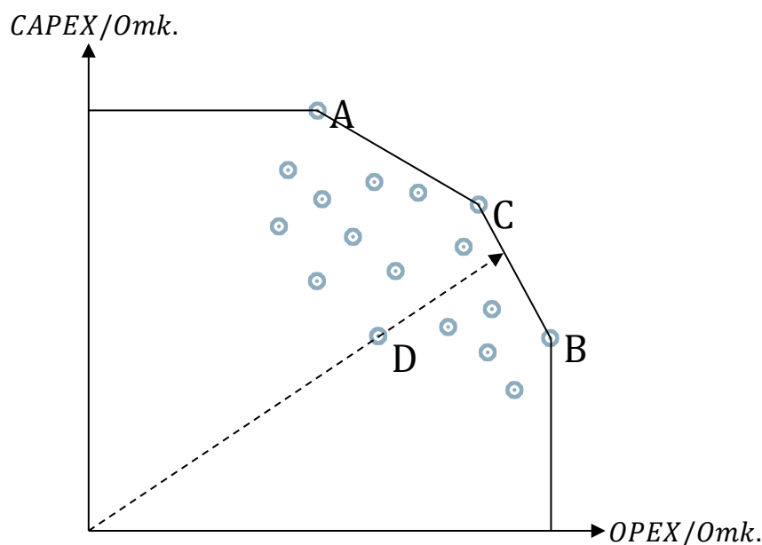
Figur 2.1 Illustrativt eksempel af DEA
