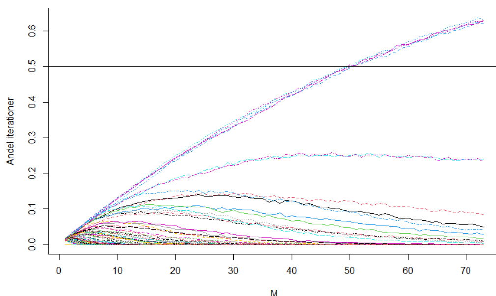
Figur 3.6 Andel af iterationer et selskab indgår på fronten
