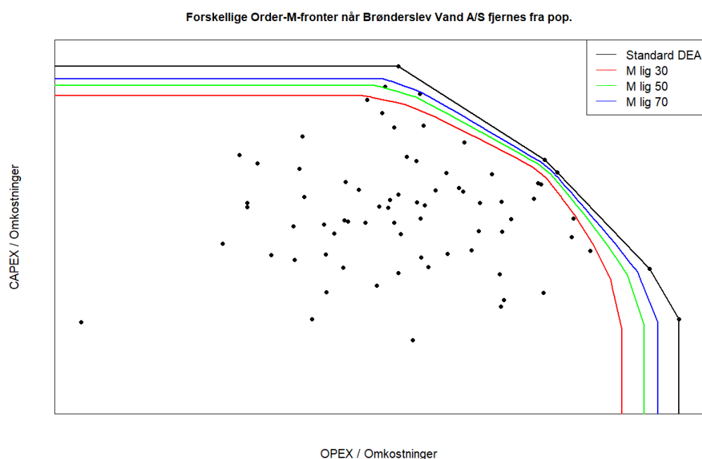
Figur 3.5 Sammenligning af fleksibiliteten af fronten i DEA og Order-M
